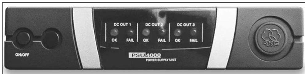
Fig 1: Elementos de mando y LEDs de control en el panel frontal
