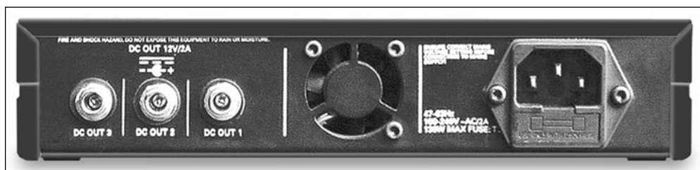
Fig. 2: Entradas y salidas en el panel posterior
