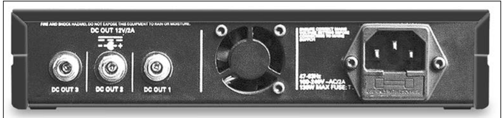
Fig. 2 : Entrées et sorties en face arrière
